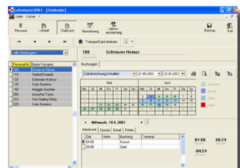
Übersicht ZeitAssist
