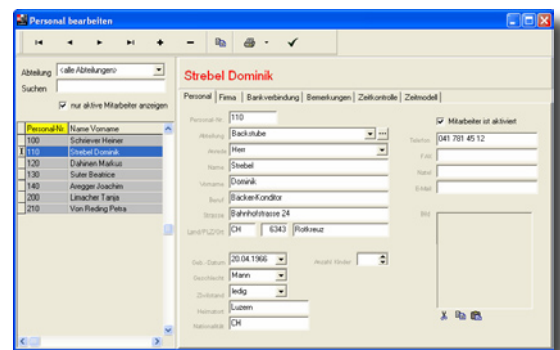
Stammdaten erfassen
